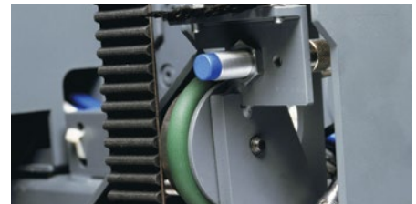
Vigilancia de la tensión de la correa de transmisión
