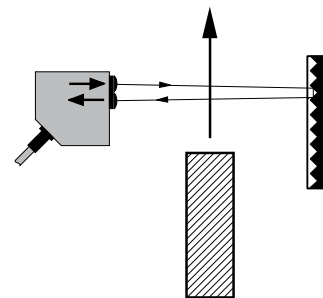
Fig. 10: Detección con sensores reflex
