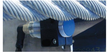
Control de distancia para control de posición
